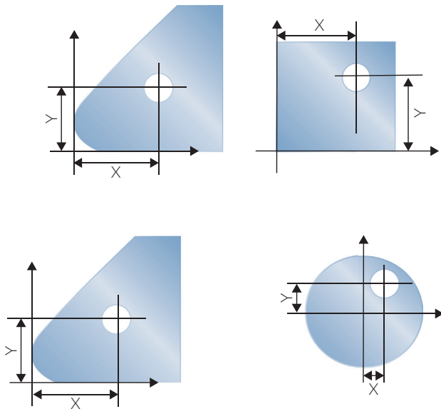
Abb. 11: Bohrlochlage
