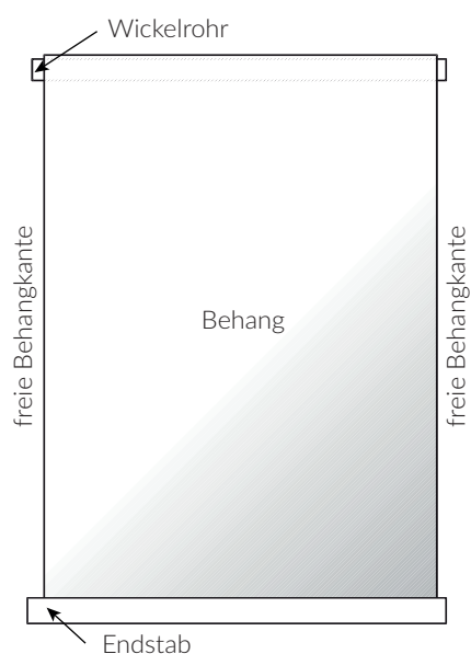
Abb. 54: Zulässige Einrollung
