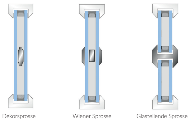
Abb. 35: Sprossenarten
