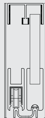
Robustus-Beschlag mit seitlichem Rahmenprofil
