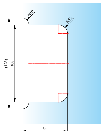
Glasbearbeitung 3 mm Luft glass processing 3 mm gap
