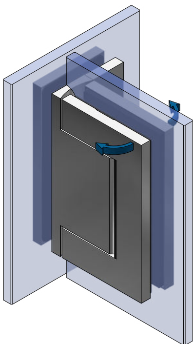
ohne Dichtprofil, Glasbearbeitung für 8 mm without sealing profile, glass processing for 8 mm
