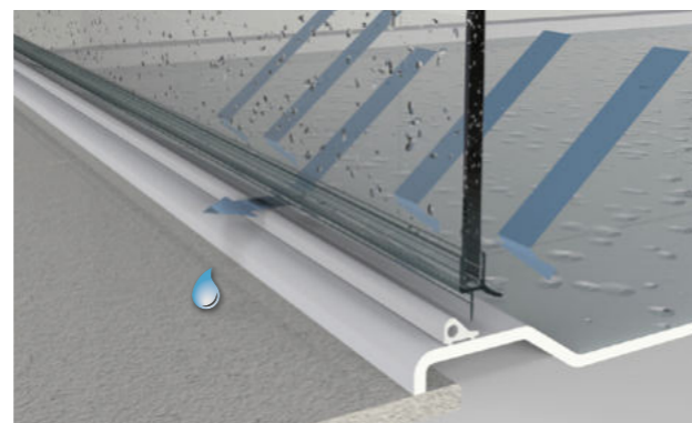
mit Dichtprofil und Schwallenschutz - Kaum Wasser kann nach aussen dringen.
