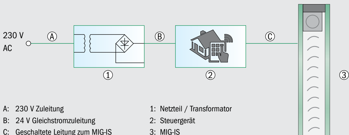
Bild 11: Darstellung Grundanschluss
