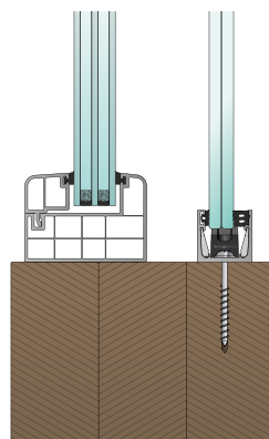
Holz-Rahmen
