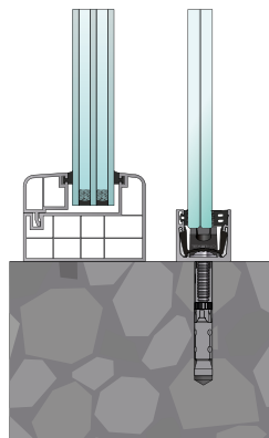
Stein-Rahmen
