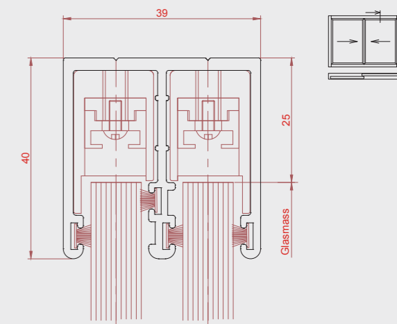
exemplarisch 2-gleisige Schnittzeichnungen Boden- und Deckenschiene
