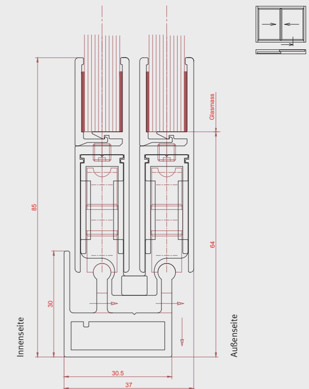
exemplarisch 2-gleisige Schnittzeichnungen Boden- und Deckenschiene
