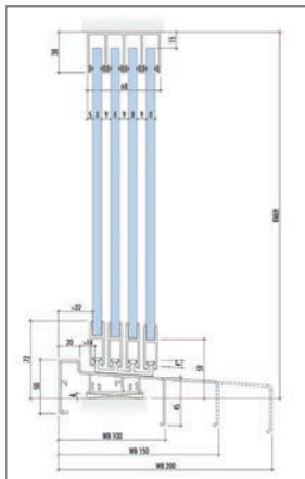
Abb. 8.51: Systemschnitt
