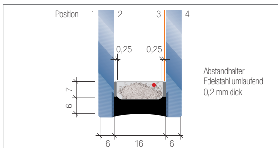
Abb. 3.2: Isolierglas-Aufbau
