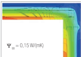
Abb. 3.11: Isothermen-darstellung [1]
