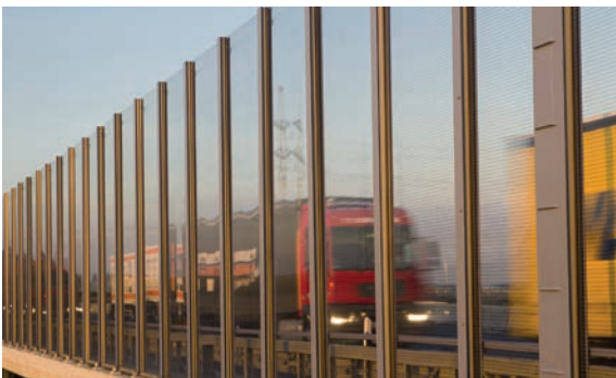
Abb. 5.6: Straßeneinhausung
