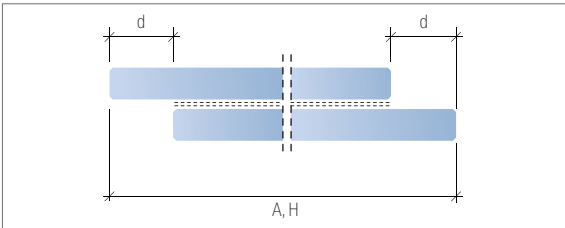
Abb. 2.21: Kantenversatz bei VSG (d)
