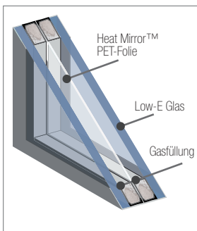
Abb. 4.14: Heat Mirror™ Schematische Darstellung
