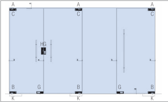
Abb. 8.55: Beispiel Ganzglasanlage mit Oberlicht
