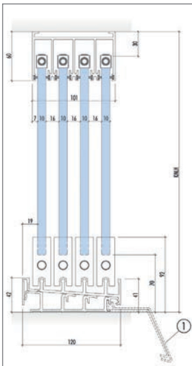
Abb. 8.52: Systemschnitt
