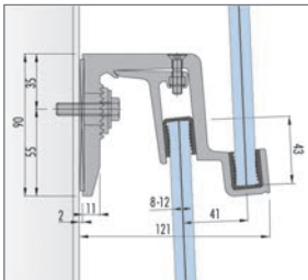
Abb. 8.30: Systemschnitt Mitte
