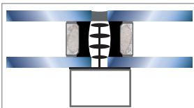
Abb. 3.20: Variante 3 a: Stoßfuge (2-fach IG) (Prinzipdarstellung) [1]
