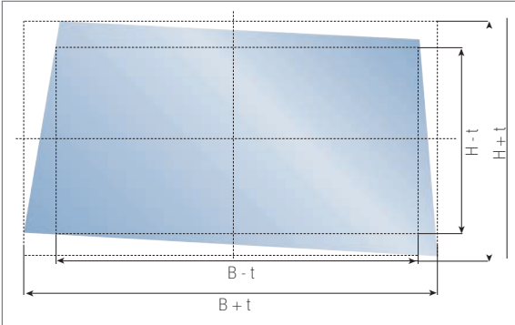
Abb. 11.19: Grenzmaße rechtwinkliger Scheiben
