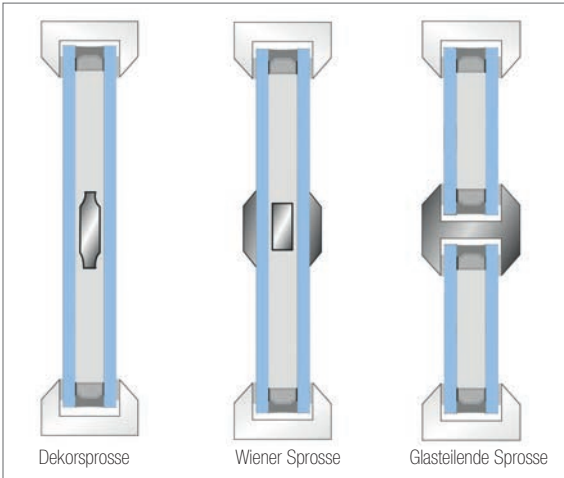
Abb. 11.23: Sprossenarten
