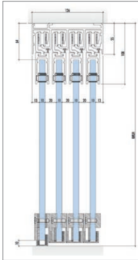
Abb. 8.45: Systemschnitt
