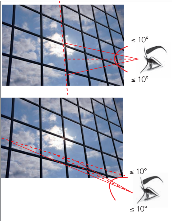
Abb. 11.22: Beschränkung der Betrachtungswinkel bei der Beurteilung der farblichen Homogenität einer Fassade
