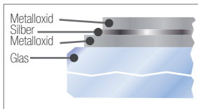
Abb. 4.1: Edelmetallbeschichtung
