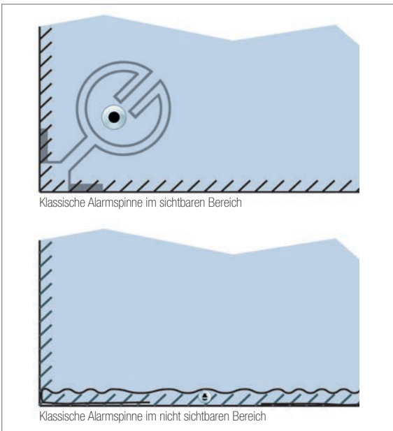
Abb. 2.10: Varianten der Leiterschleifen (Spinne)
