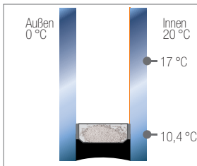
Abb. 4.4: Aluminium-Abstandhalter
