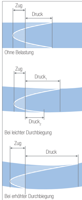
Abb. 2.4: Spannungsverteilung
