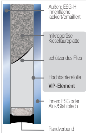
Abb. 4.16: Vakuum-Paneel
