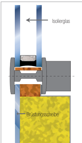
Abb. 6.9: Warmfassade (Systemschnitt)
