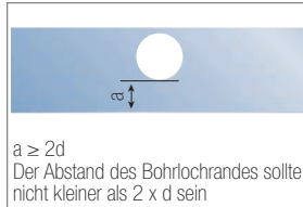
Abb. 11.12: Lage des Bohrlochs zur Ecke
