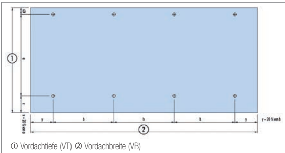
Abb. 8.7: Montageansicht / Glasbohrung
