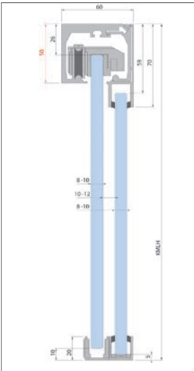
Abb. 8.37: Taschenmontage
