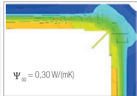
Abb. 3.25: Isothermendarstellung [1]
