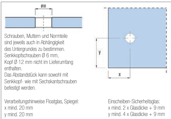
Abb. 8.20: Technischer Aufbau
