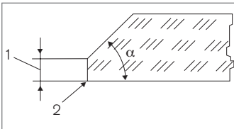
Abb. 11.5: Gehrungskante
