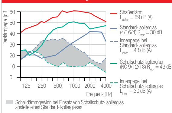
Abb. 5.1: Vergleich Schalldämmung Standard- / Schallschutz-Isolierglas
