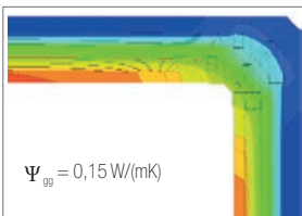
Abb. 3.19: Isothermen-darstellung [1]
