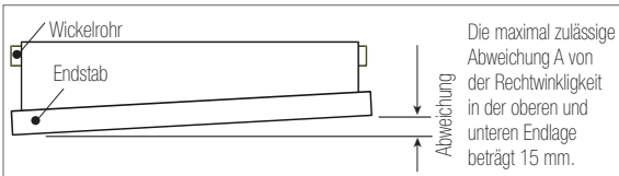
Abb. 11.39: Zulässige Abweichung der Rechtwinkligkeit
