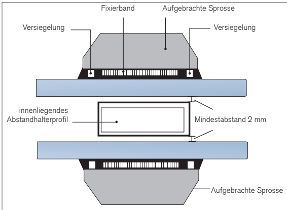
Abb. 10.4: Beispiel für Wiener Sprosse
