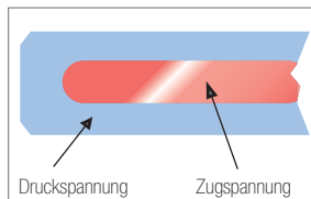
Abb. 2.2: Spannungsgefüge
