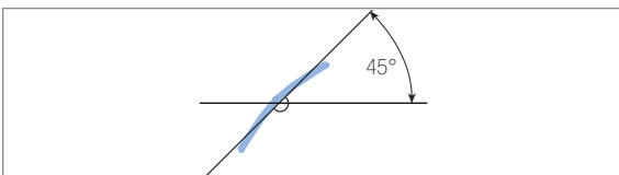
Abb. 11.37: Schwenkbarkeit der Lamellen (einseitig schließend)
