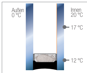
Abb. 4.5: „warm edge“-Abstandhalter
