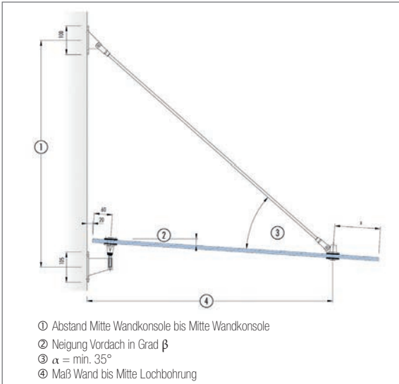
Abb. 8.3: Montageansicht
