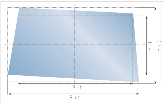
Abb. 11.16: Grenzabmaße für rechteckige Scheiben
