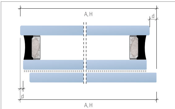
Abb. 2.22: Kantenversatz bei Isolierglas (d)
