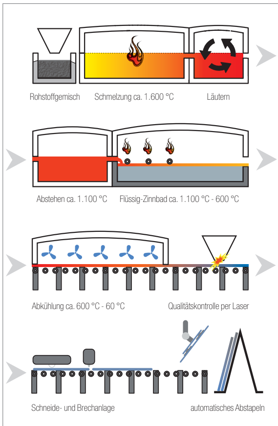
Abb. 1.1: Floatglasherstellung (Schematische Darstellung)
