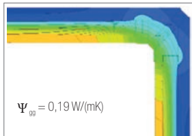
Abb. 3.17: Isothermendarstellung [1]
