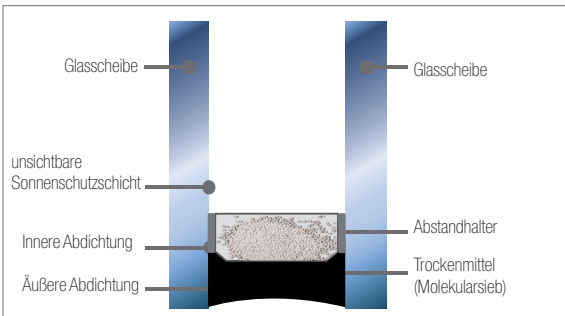
Abb. 6.1: Sonnenschutzglas-Aufbau
