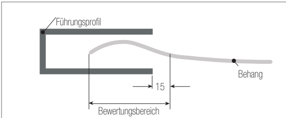
Abb. 11.44: Faltenbreite
