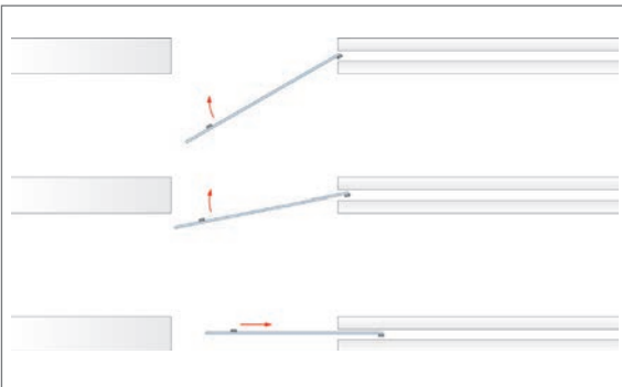
Abb. 8.37: Taschenmontage
