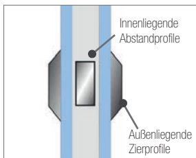
Abb. 3.36: Wiener Sprosse
