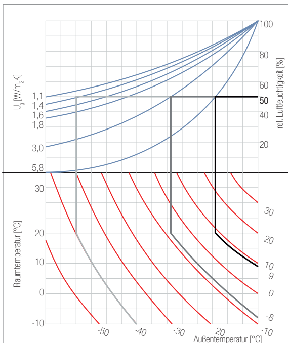
Abb. 3.32: Taupunkt diagramm (nach DIN 4701)
