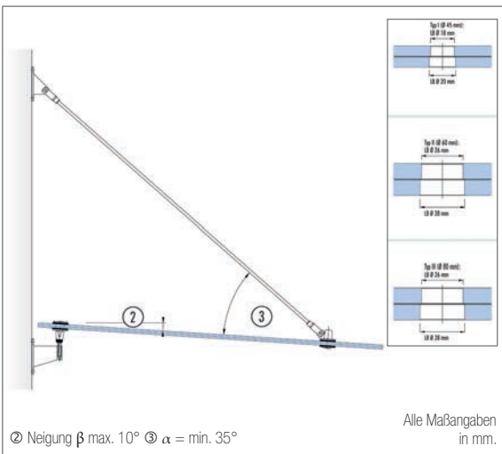
Abb. 8.7: Montageansicht / Glasbohrung
