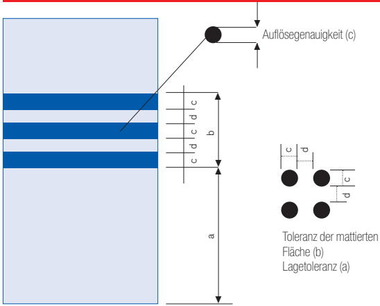
Abb. 2.11: Lage- und Designtoleranzen der Abmessung bei teilmattierten Flächen
