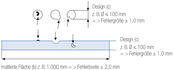
Abb. 2.12: Geometrie des Designs - Designfehler
