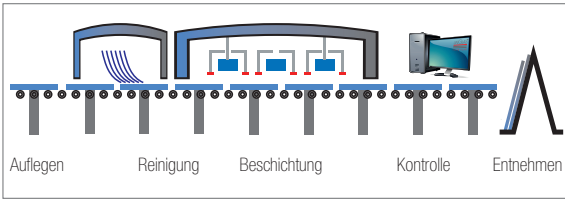
Abb. 4.2: Magnetron-Verfahren (Schematische Darstellung)
