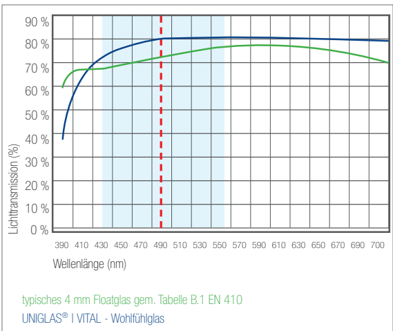
Abb. 4.13: Vergleich der Lichttransmission im wichtigen Wellenbereich von 460 nm zwischen einem 4 mm Floatglas nach Norm und dem neuen UNIGLAS® I VITAL Wohlfühlglas
