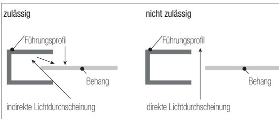
Abb. 11.40: Lichtdurchscheinungen
