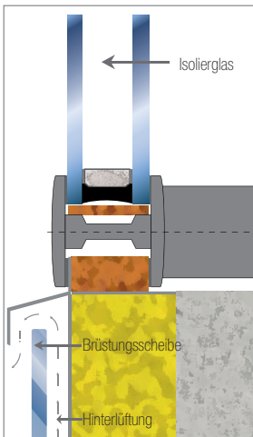
Abb. 6.10: Kaltfassade (Systemschnitt)
