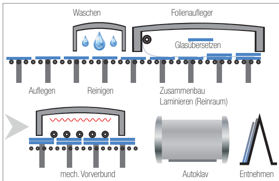
Abb. 2.28: Herstellung Verbund-Sicherheitsglas
