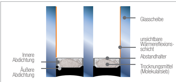
Abb. 4.3: Dreischiebiger Isolierglas-Aufbau
