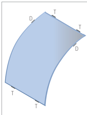
Abb. 2.26: Anordnung der Klotzung bei System 2
