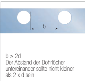
Abb. 11.11: Lage benachbarter Bohrlöcher
