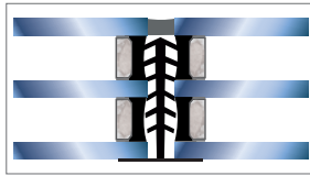
Abb. 3.14: Variante 2 b: Stoßfuge (3-fach IG) (Prinzipdarstellung) [1]
