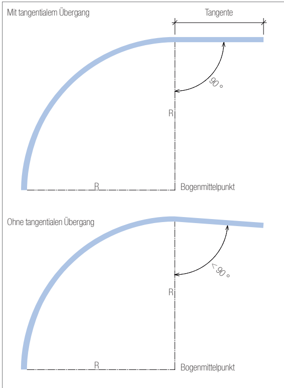
Abb. 2.24: Tangentiale Übergänge
