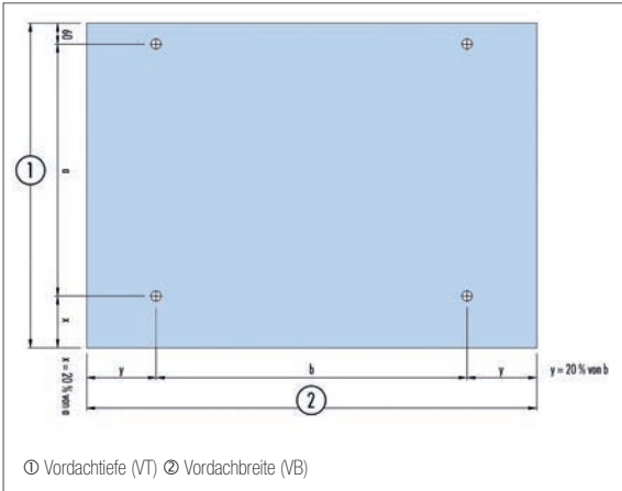
Abb. 8.4: Bohrlochvorlage
