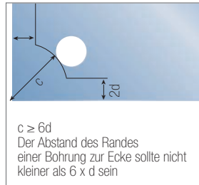
Abb. 11.12: Lage des Bohrlochs zur Ecke
