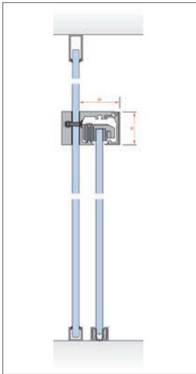
Abb. 8.36: Systemschnitt
