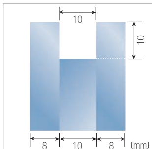
Abb. 11.18: Stufen VSG
