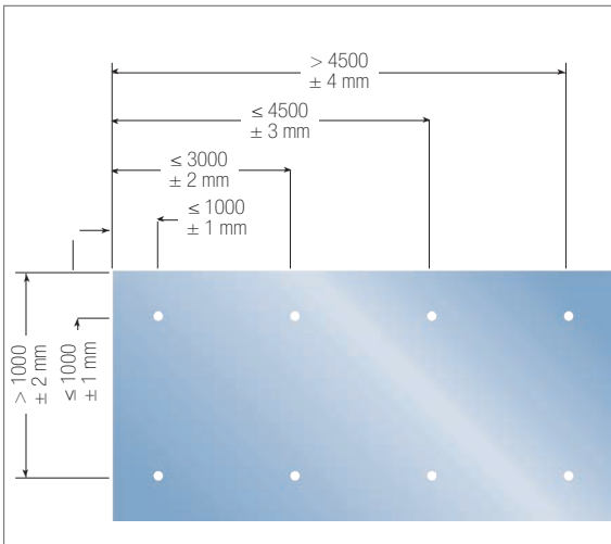
Abb. 11.14: Lochbohrungslagen
