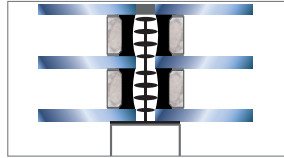
Abb. 3.22: Variante 3 b: Stoßfuge (3-fach IG) (Prinzipdarstellung) [1]
