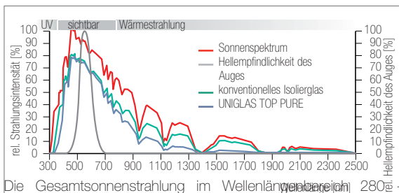
Abb. 3.28: Globalstrahlung
