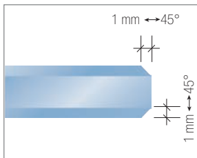
Abb. 11.6: Kantenbearbeitung
