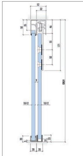
Abb. 8.42: Systemschnitt
