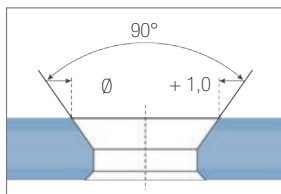
Abb. 11.8: Senklochabmaß
