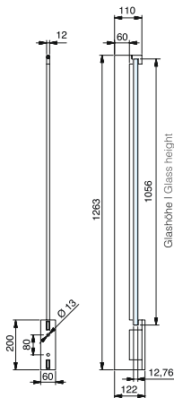
Einzelpfosten für Frontmontage
