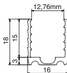
Gummiprofil
