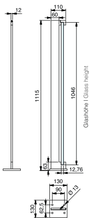
Einzelpfosten für Aufsatzmontage
